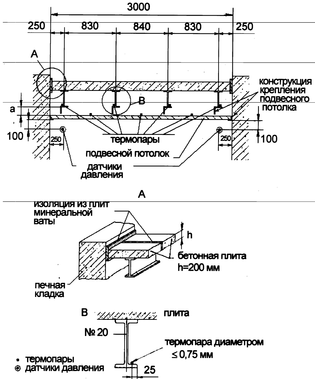
Рисунок А.1 — Схема испытательного блока
