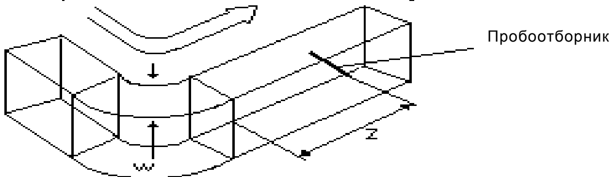
Рисунок 1 : Расположение извещателей в воздушных каналах
