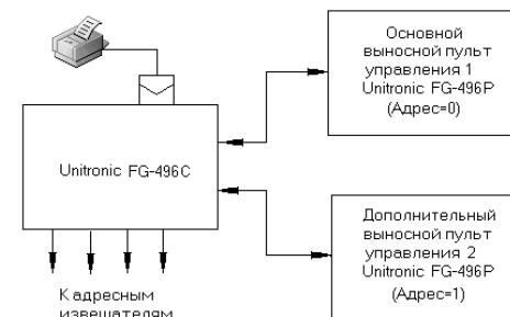
Рис. 4. Схема подключения контроллера с двумя выносными пультами управления
