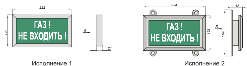
Оповещатель световой «Гамма-01 ОС».
