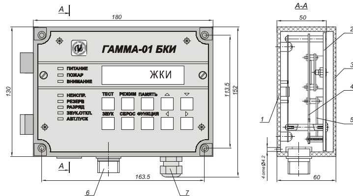
Блок клавиатуры и индикации «Гамма-01 БКИ»: 1 - корпус; 2 - панель; 3 - крышка; 4 - плата; 5 - плата; 6 - вилка 2PM22B10Ш1B1; 7 - гермоввод.
