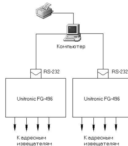
Рис. 5. Схема объединения АПКП в сеть с управлением от компьютера с помощью интерфейса RS-232
