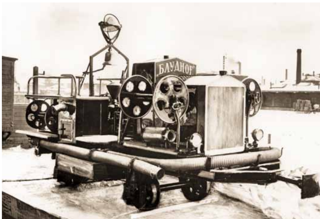
Пожарная машина на железнодорожной платформе. Ленинград. 1928 г.
