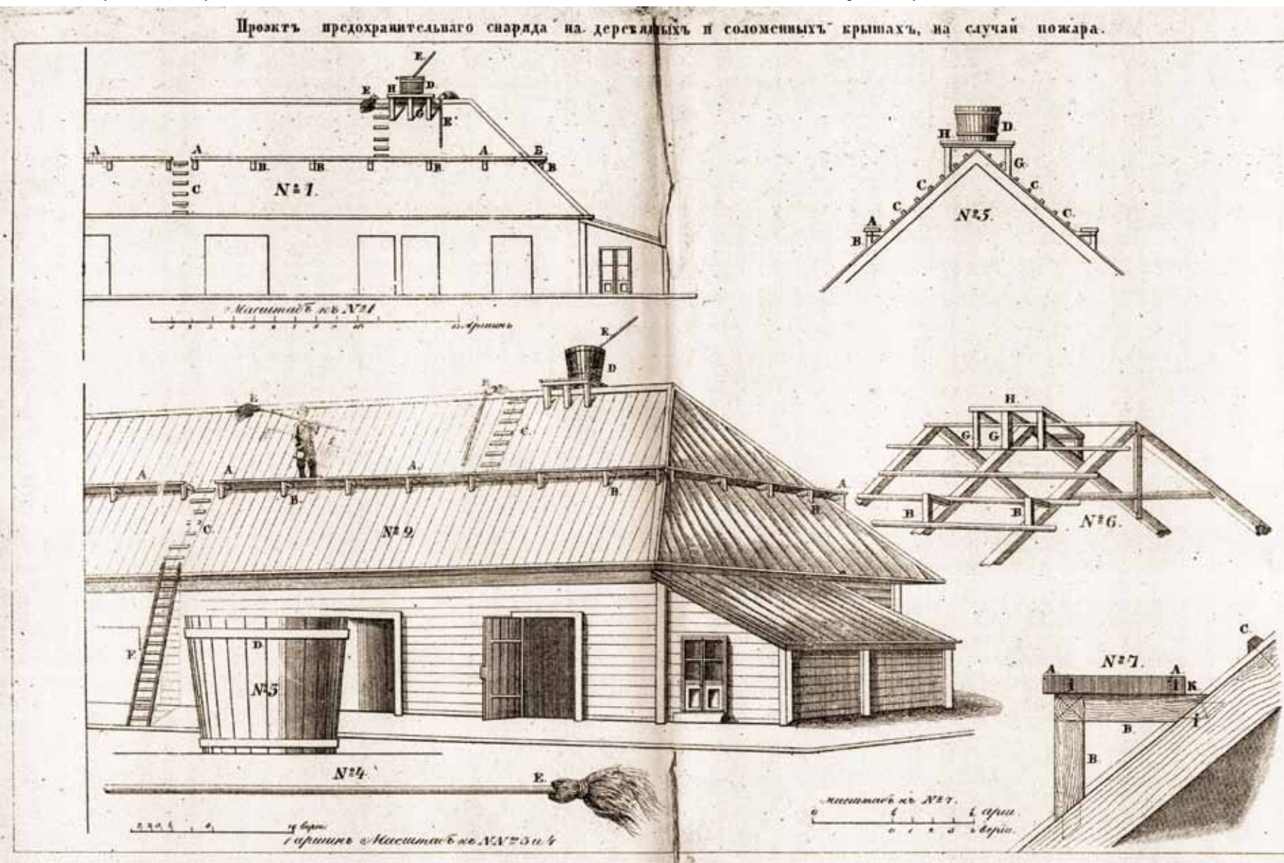
Проект предохранительнаго снаряда на деревянныхъ и соломенныхъ крышахъ, на случай пожара. 1849 г. ЦГИА СПб. Ф.697. Оп.2. Д.68. Л.6 A preventive shell plan on wooden and straw roofs, in case of a fire. 1849. Central State Historical Archives. Saint-Petersburg. F.697. Op.2. D.68. L.6
