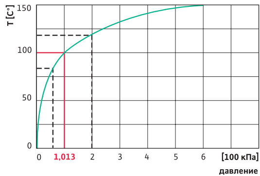
Температура кипения воды как функция давления
