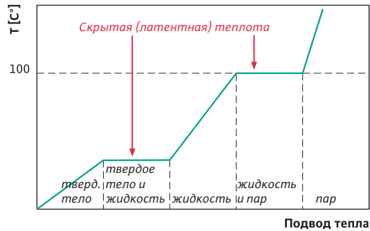
Изменение агрегатного состояния при повышении температуры
