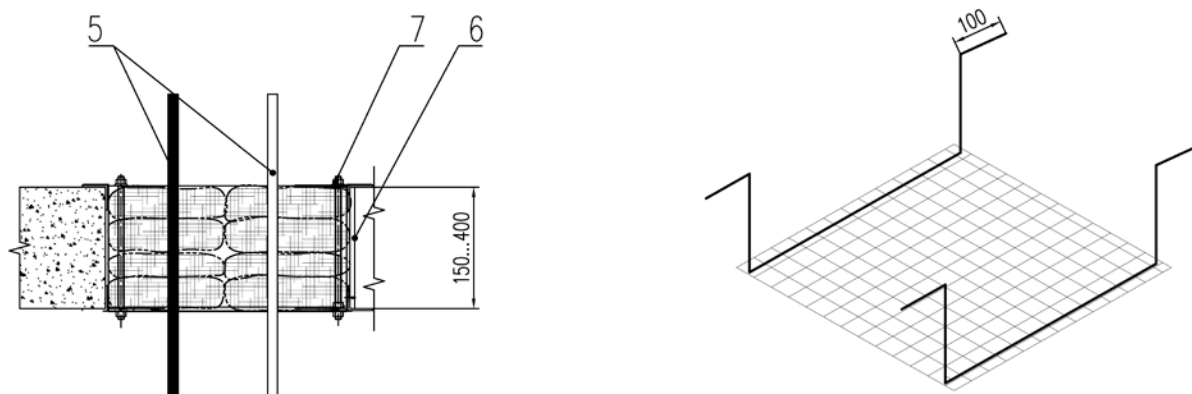
Рис. 17 Горизонтальное исполнение с биндажом.
