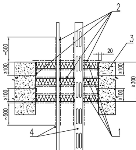
Рис. 2. Горизонтальное исполнение.
