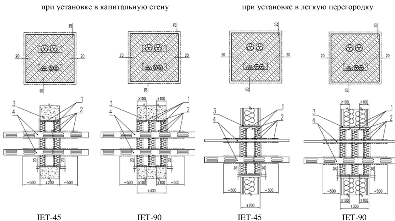
Рис. 1. Вертикальное исполнение.
