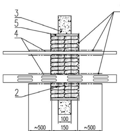
Рис. 7. Проходка с наращиванием толщины стены
