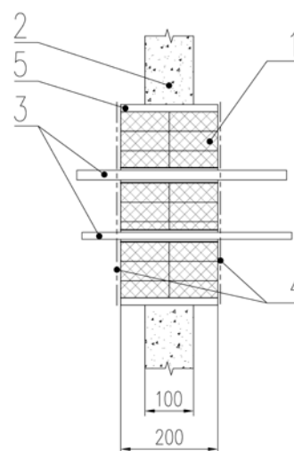
Рис. 11. Проходка с наращиванием толщины стены.
