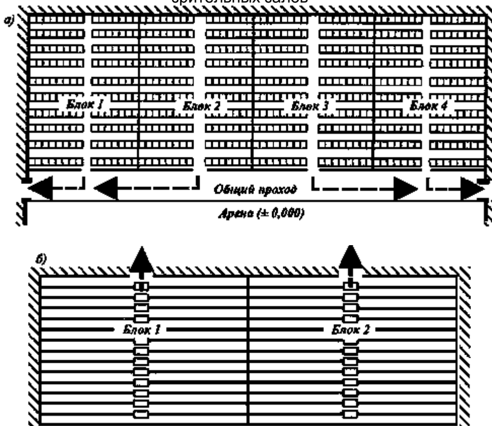
а - при эвакуации в общий горизонтальный проход на уровне арены; б - при эвакуации вверх через дверной проем или на горизонтальный участок Рисунок И.2 - Схемы разделения мест на блоках на трибунах спортивно-зрелищных и универсальных залов при расположении люков
