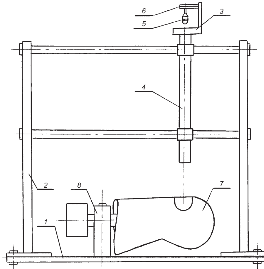
1 — станина; 2 — стойки; 3 — держатель; 4 — направляющая труба; 5 — ударник; 6 — спусковое устройство; 7 — испытываемое средство защиты; 8 — устройство для закрепления испытываемого средства защиты
