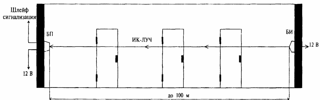
Рисунок 6.14- Блокировка дверей (ворот) на открывание извещателями активными линейными опико-электронными
