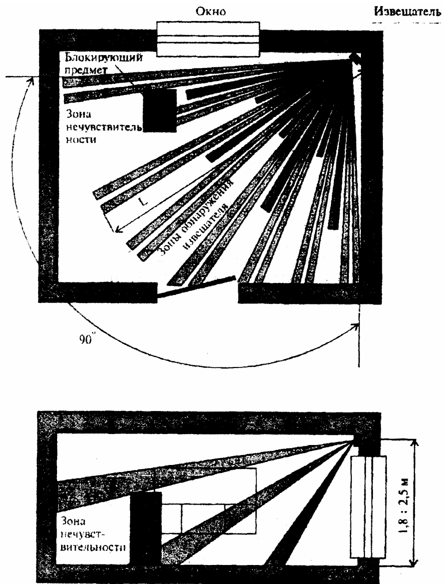
Рисунок 6.44 - Одновременная блокировка объема и отдельных предметов объемными пассивными оптико-электронными извещателями
