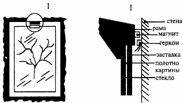
Рисунок 6.41 - Блокировка отдельных предметов магнитоконтактными извещателями
