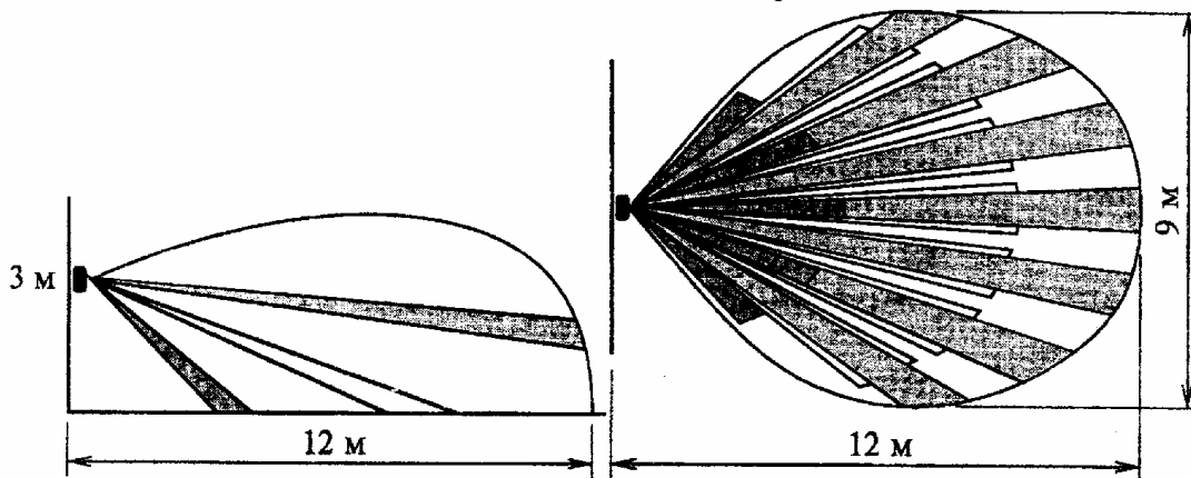
Рисунок 3.57 - Извещатель "Сокол-1"
