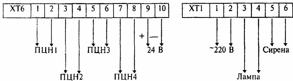
Рисунок 4.23 - "Рубин-6"
