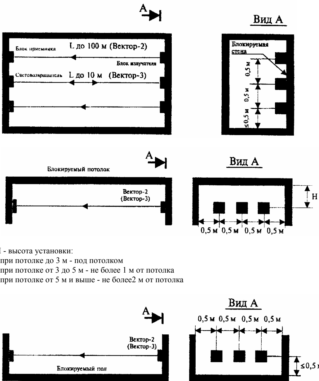
Рисунок 6.27 - Блокировка стен, потолка и пола на проникновение извещателями активными линейными оптико-электронными
