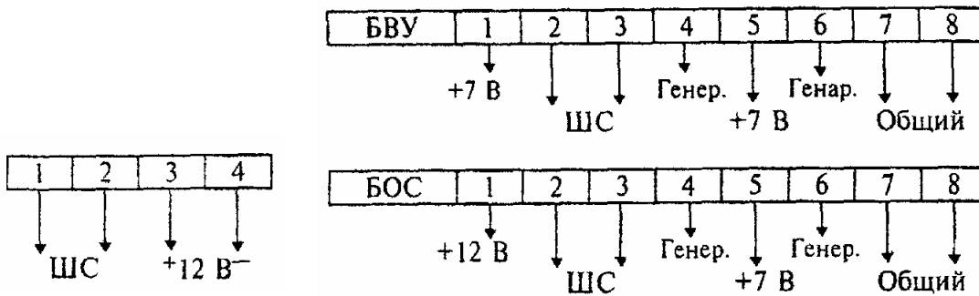
Рисунок 3.19 - "Стекло-1"
