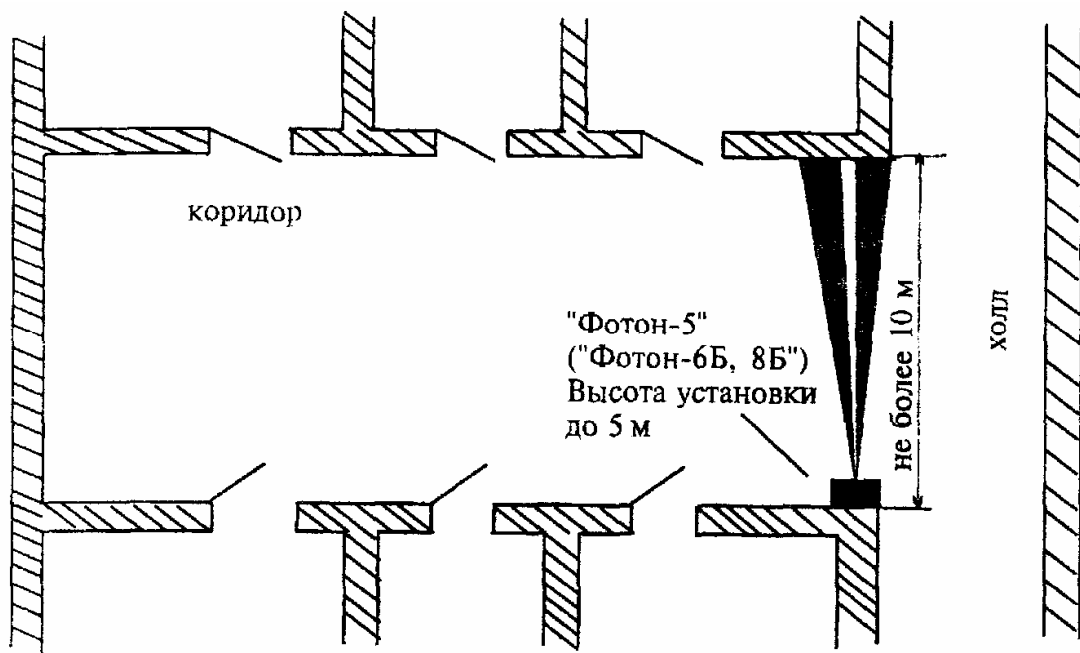
Рисунок 6.39 - Блокировка коридора извещателями пассивными опто-электронными с зоной обнаружения типа "занавес"
