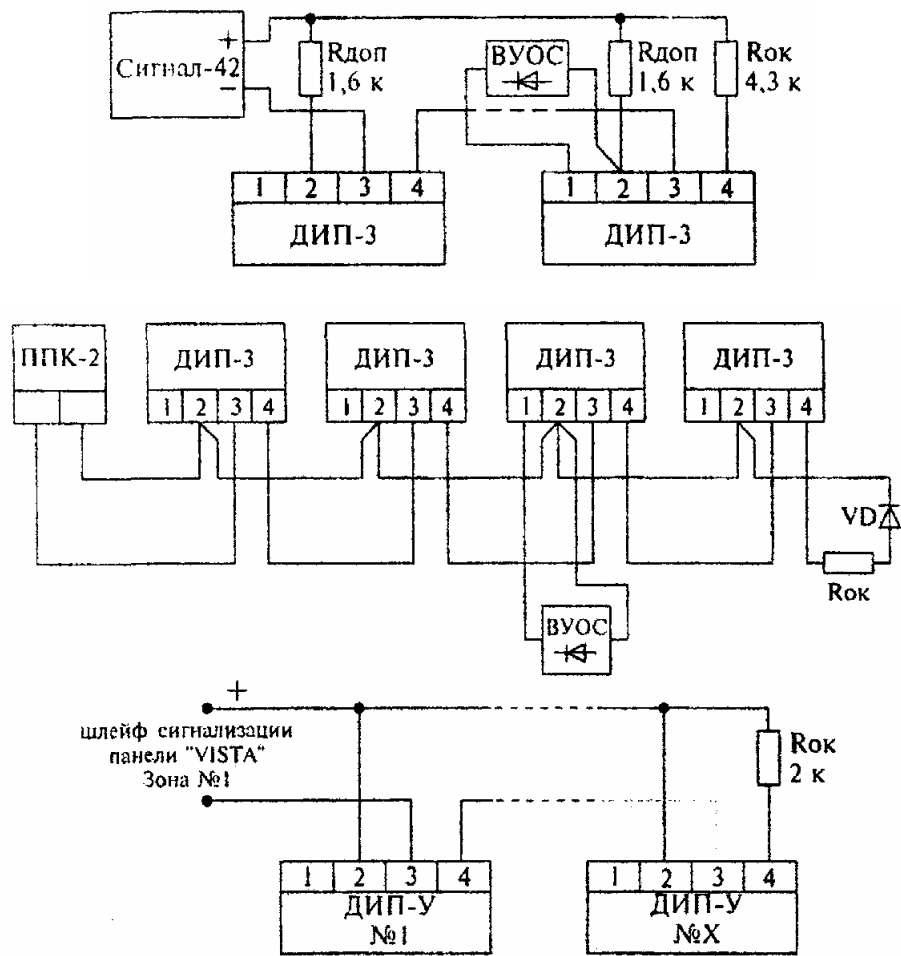
Рисунок 7.6 - Извещатель типа ИП 212-5 "ДИП-3"
