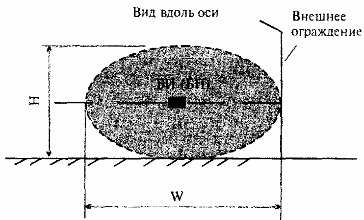
Рисунок 6.46 - Блокировка внешнего ограждения извещателем радиоволновым "Радий-1" ("Радий-2")
