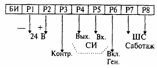
Рисунок 3.37 - "Вектор-СПЭК"
