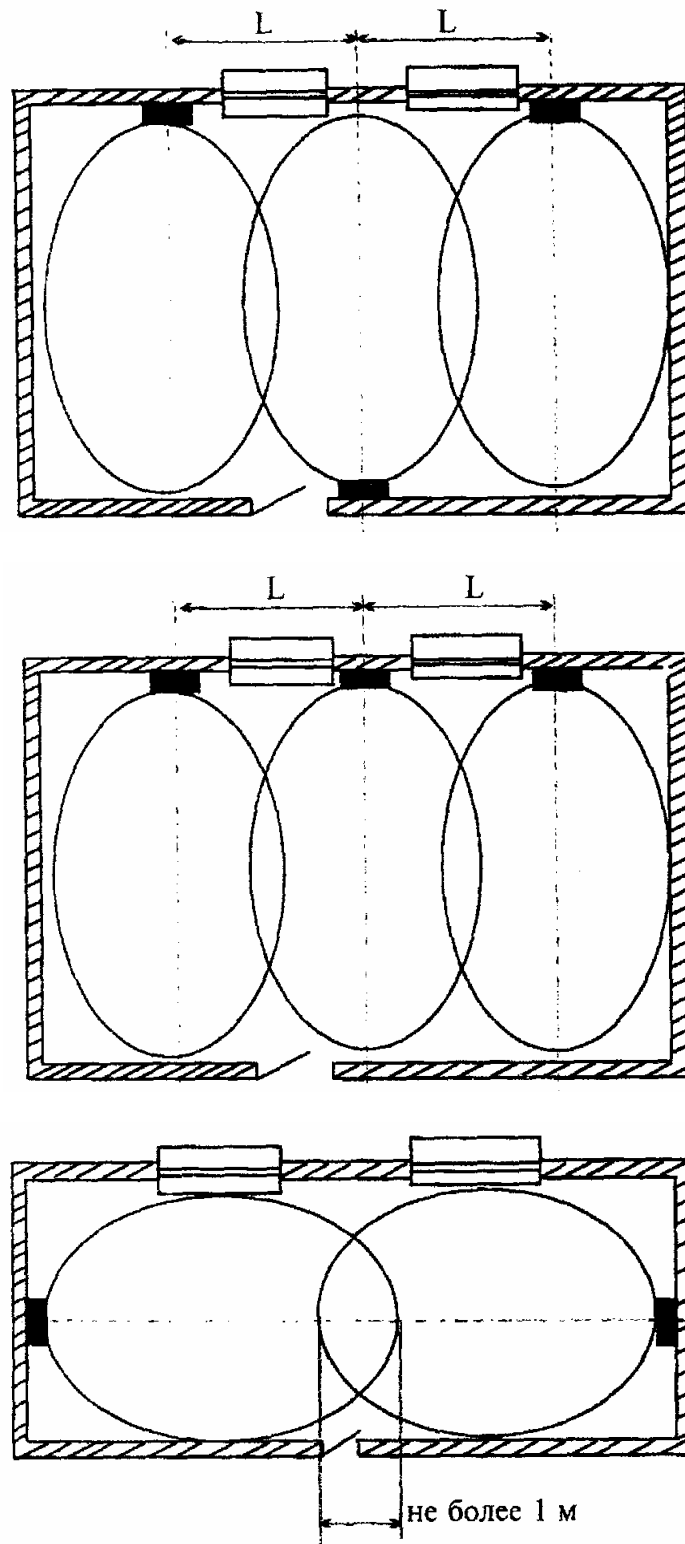
Рисунок 6.30 - Блокировка помещения несколькими радиоволновыми, ультразвуковыми и комбинированными извещателями
