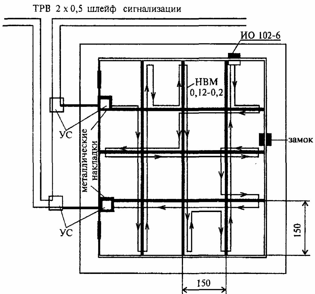
Рисунок 6.21 - Блокировка оконных решеток, решеток воздухопроводов и решетчатых дверей проводом
