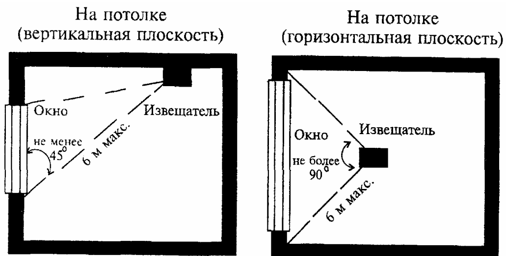
Рисунок 6.3 - Блокировка двухстворчатого окна извещателями магнитоконтактными и поверхностными ударноконтактными
