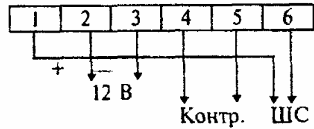
Рисунок 3.30 - "Гюльпан-3"
