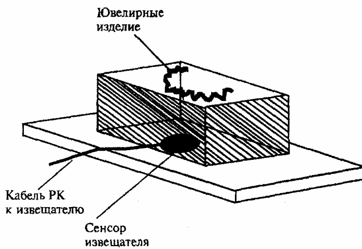
Рисунок 6.43 - Блокировка отдельных предметов извещателем поверхностным пьезоэлектрическим "Гюрза-050М"
