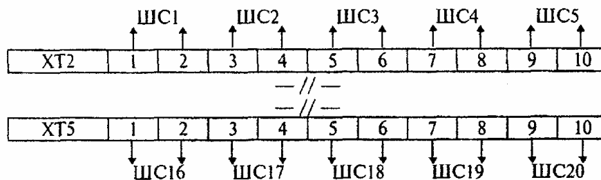
Рисунок 4.22 - "Рубин-3"
