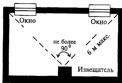
Рисунок 6.4 - Варианты установки извещателя охранного поверхностного "Стекло-1"
