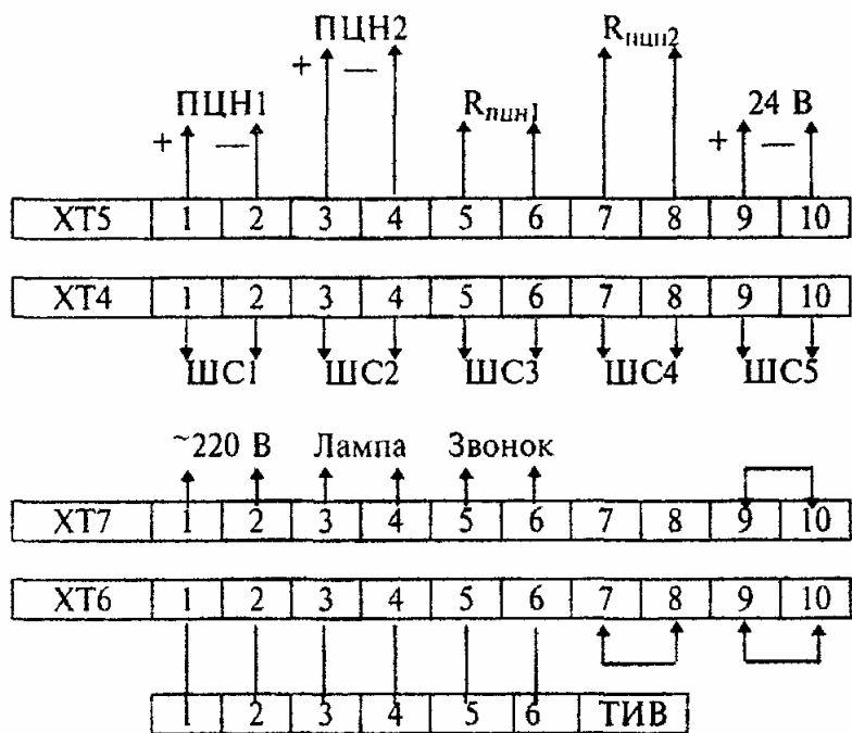
Рисунок 4.19 - "Квинта"
