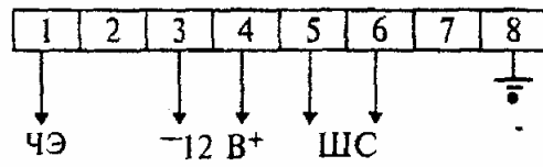
Рисунок 3.17- "Пик"
