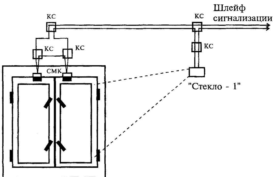
Рисунок 6.4 - Варианты установки извещателя охранного поверхностного "Стекло-1"
