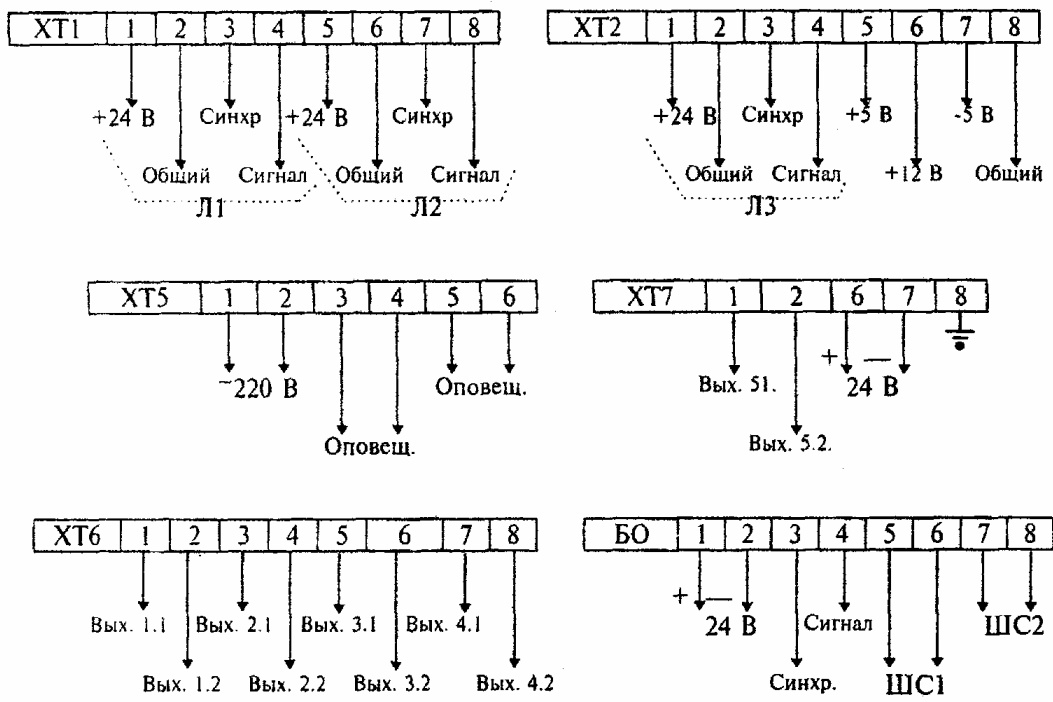
Рисунок 4. 27 - "Буг"
