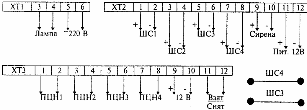
Рисунок 4.17 - "Сигнал-ВК-4"
