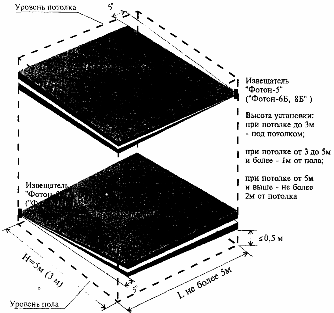
Рисунок 6.24 - Блокировка стен, потолка и пола на проникновение извещателями пассивными опико-электронными с зоной обнаружения типа " занавес ".
