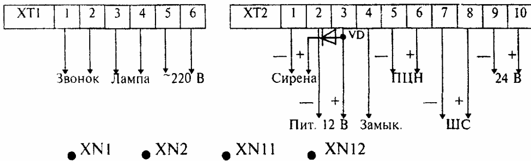
Рисунок 4.17 - "Сигнал-ВК-4"
