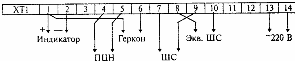
Рисунок 4.12 - "Сигнал-41"
