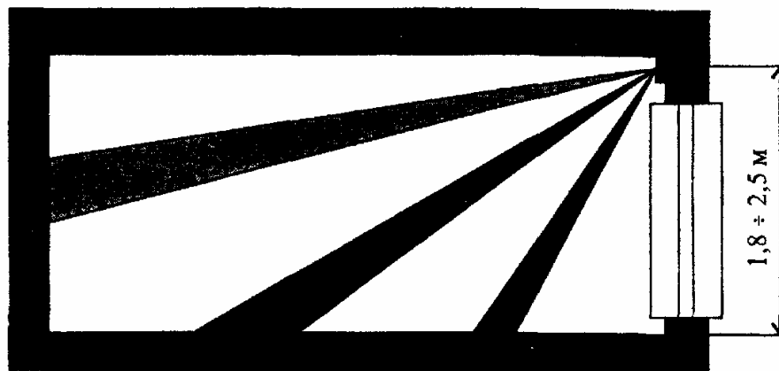
Рисунок 6.28 - Одновременная блокировка на проникновение стен, пола и потолка, а также объема помещения объемными пассивными опико-электронными извещателями
