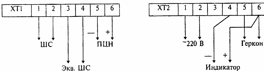
Рисунок 4.13 - "Сигнал-41М"
