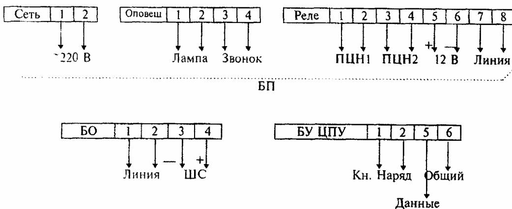
Рисунок 4. 27 - "Буг"
