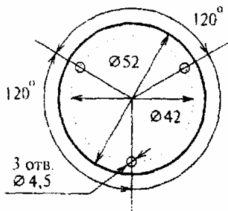
Рисунок 3.7 - "Эхо-3"
