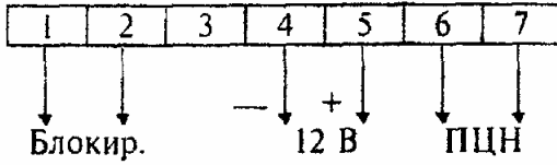
Рисунок 3.23 - "9981"
