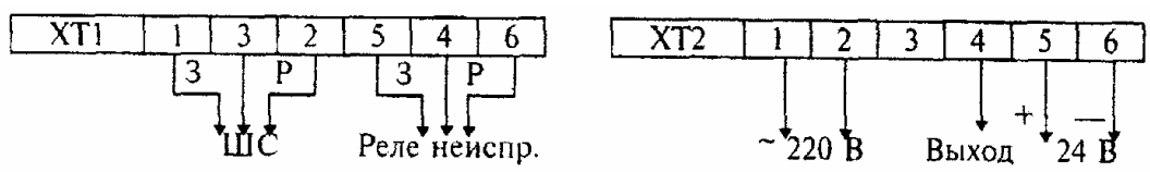
Рисунок 3.33 - "Радий-2", "Радий-2/1", "Радий-2/2"
