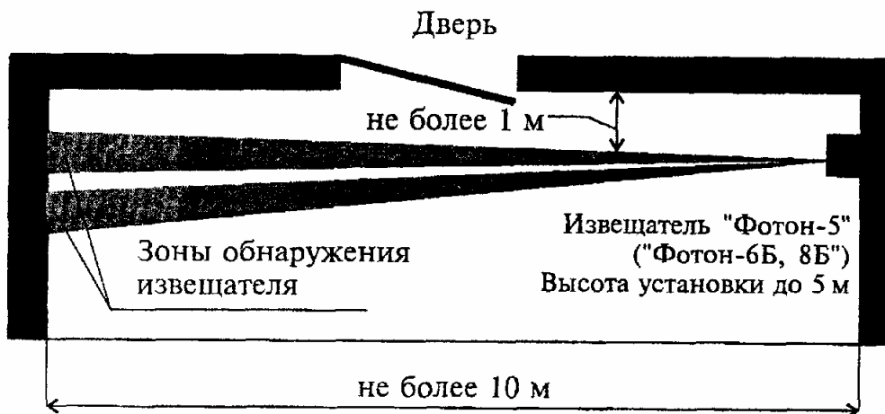
Рисунок 6.11 - Блокировка двери на проникновение извещателями пассивными оптоэлектронными с зоной обнаружения типа "занавес"
