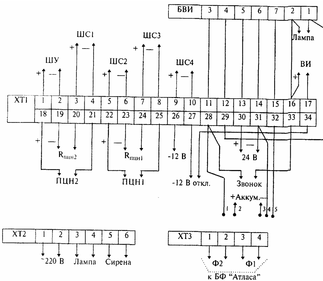
Рисунок 4.19 - "Квинта"
