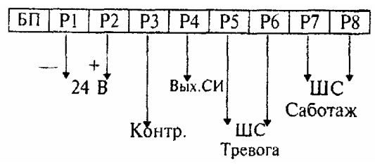
Рисунок 3.37 - "Вектор-СПЭК"
