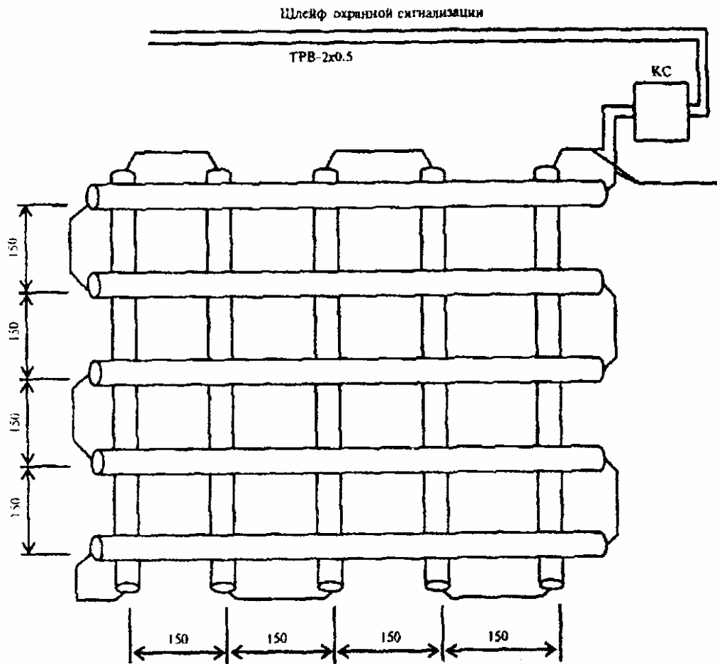
Рисунок 6.22 - Блокировка фальшрешетки воздуховода проводом
