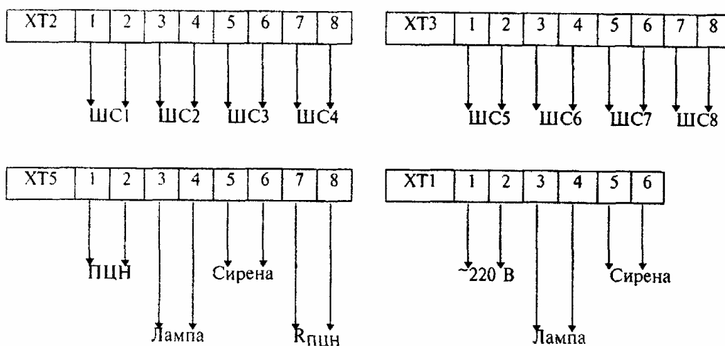
Рисунок 4.23 - "Рубин-6"
