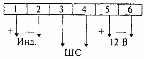
Рисунок 3.35 - "Сокол-1"
