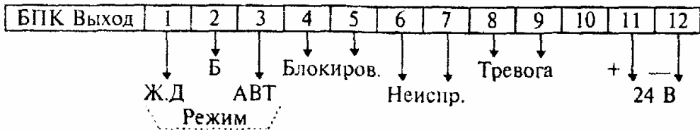
Рисунок 3.23 - "9981"
