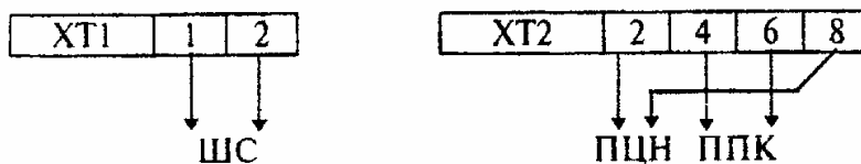
Рисунок 4.14 - "Сигнал-44"
