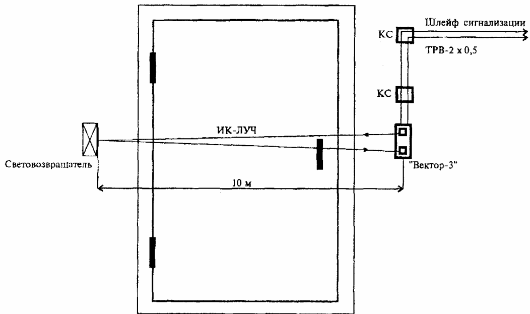
Рисунок 6.14- Блокировка дверей (ворот) на открывание извещателями активными линейными опико-электронными
