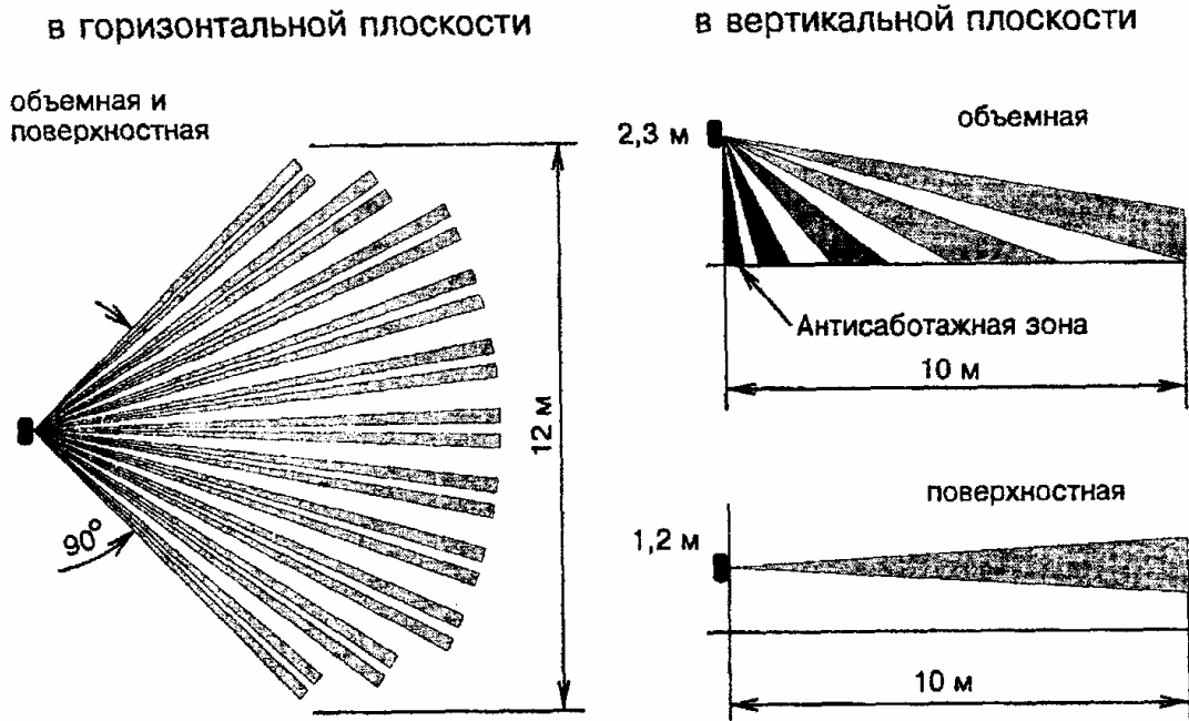
Рисунок 3.48 - Извещатель "Фотон-СК"
