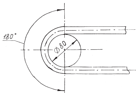
Рисунок 5 — Схема определения работоспособности воздухопроводного шланга
